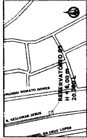
01 - PLANO DE LOCALIZAÇÃO RESERVATÓRIO 01 02 - PLANO DE LOCALIZAÇÃO RESERVATÓRIO 02 03 - PLANO DE LOCALIZAÇÃO RESERVATÓRIO 03
